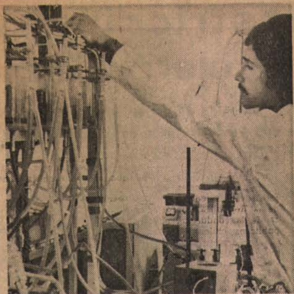
En el Instituto de Investigaciones Tecnológicas se estudia la aplicación en la minería chilena de un nuevo método para la obtención de cobre electrolítico. En la foto, la planta piloto de "Extracción por Solventes"
